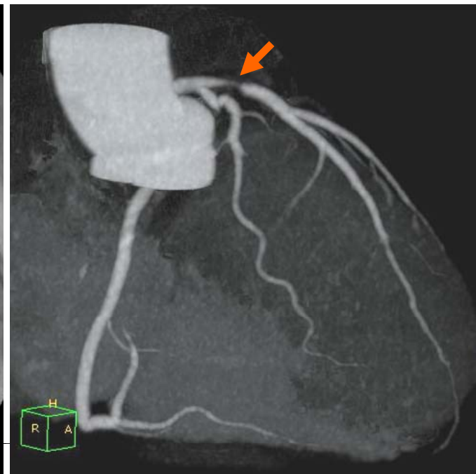
CT画像
